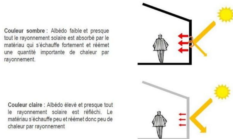
Figure 55. Incidence du rayonnement selon la couleur de la façade
