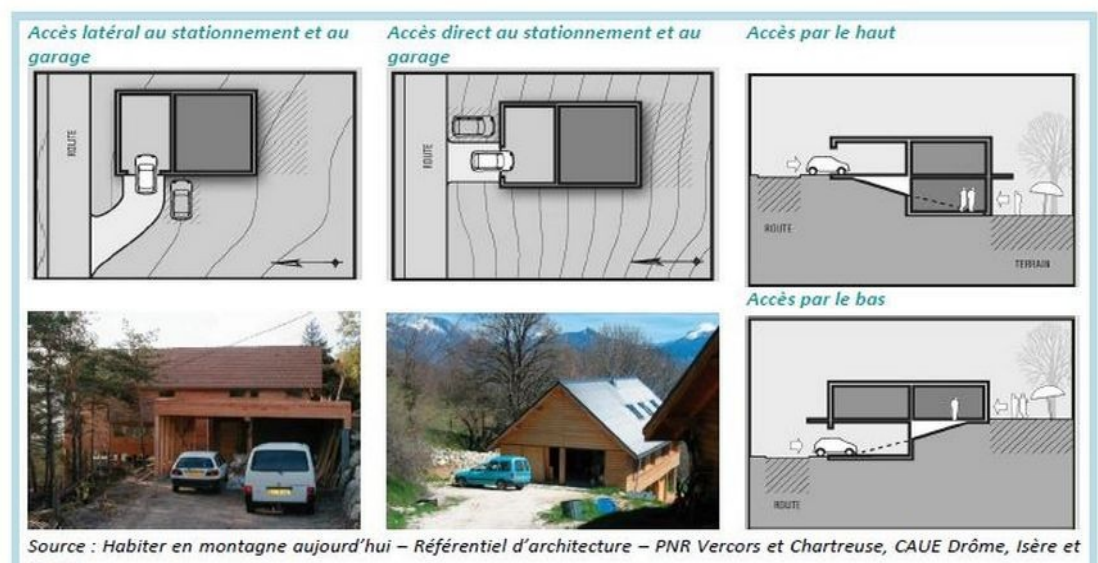
Figure 33. Diversité d'implantation de stationnement dans la pente
