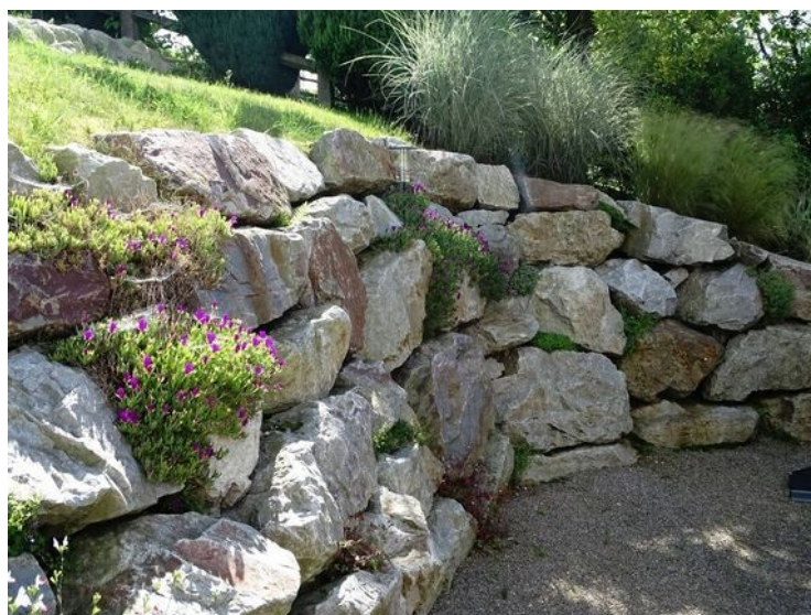
Figure 23. Exemple de mur en enrochement avec un aménagement paysager
