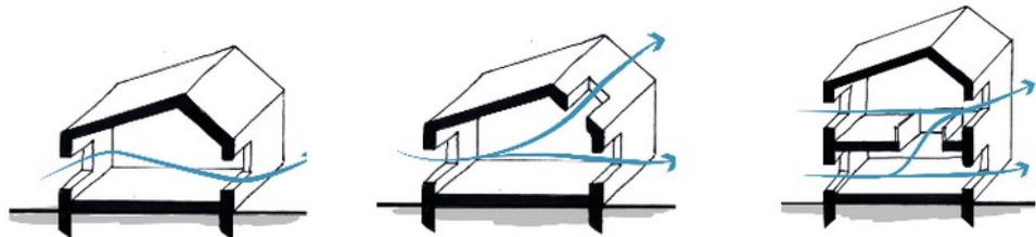
Figure 61. Diverses configurations traversantes sur plusieurs niveaux
