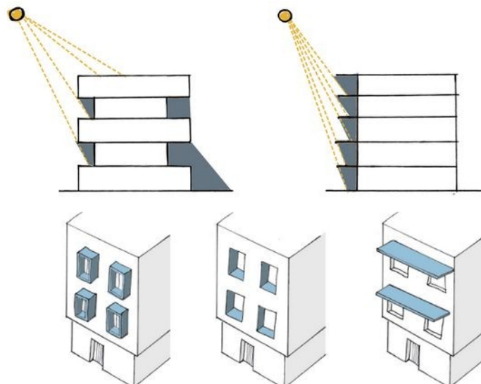
Figure 56. Schémas de principe d'un bâti qui crée ses propres ombres
