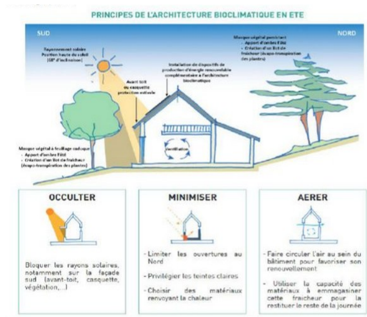
Figure 57. Principes de l'architecture bioclimatique pour le tissu pavillonnaire
