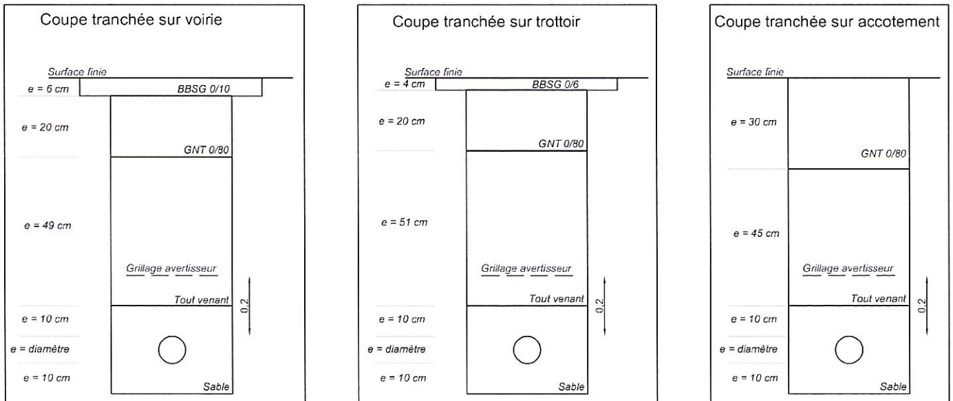
Exemple pour un fourreau/canalisation Dn90 à -85 cm
